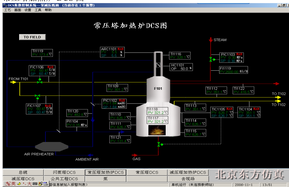
常压塔加热炉 DCS 图
