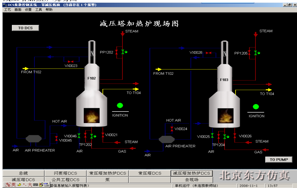
减压塔加热炉现场图
