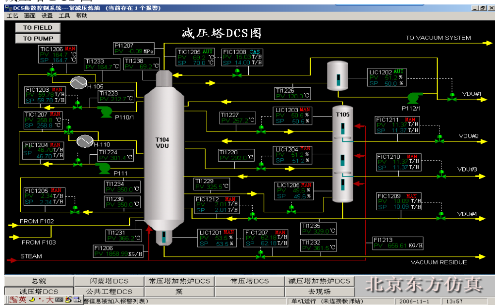
减压塔 DCS 图
