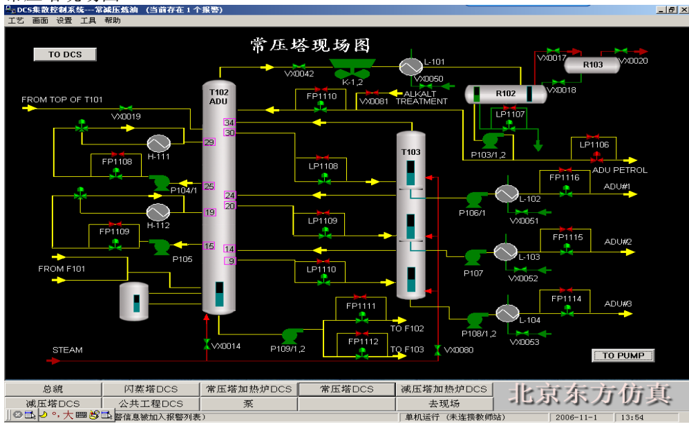
常压塔现场图
