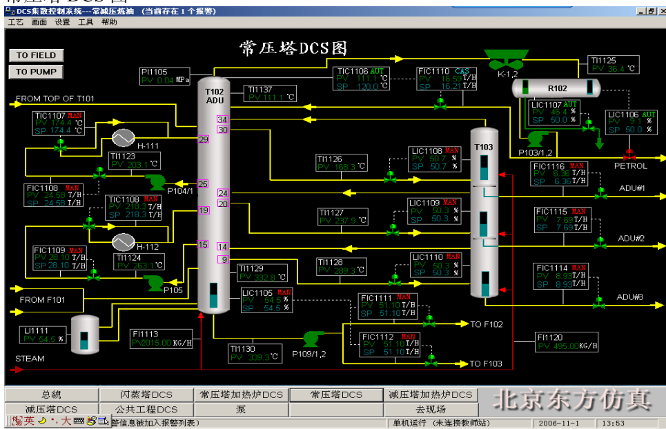
常压塔 DCS 图
