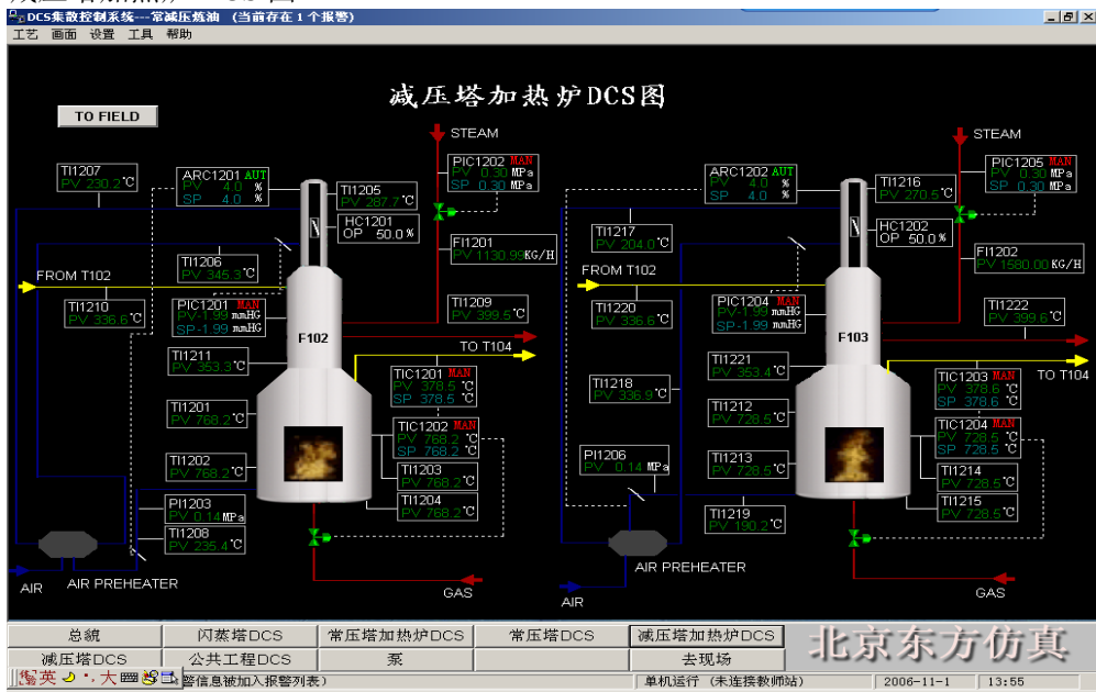
减压塔加热炉 DCS 图
